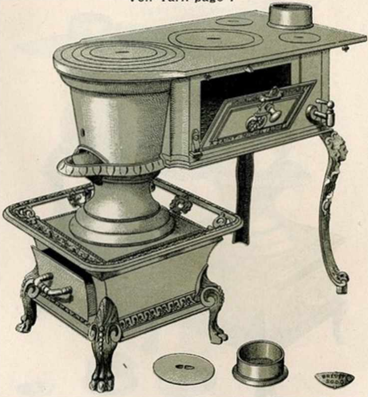
Tampon de buse mobile. Buse mobile. Papillon.
