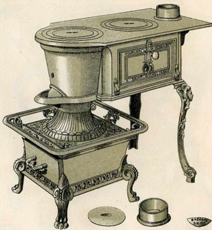
Tampon de buse mobile.
