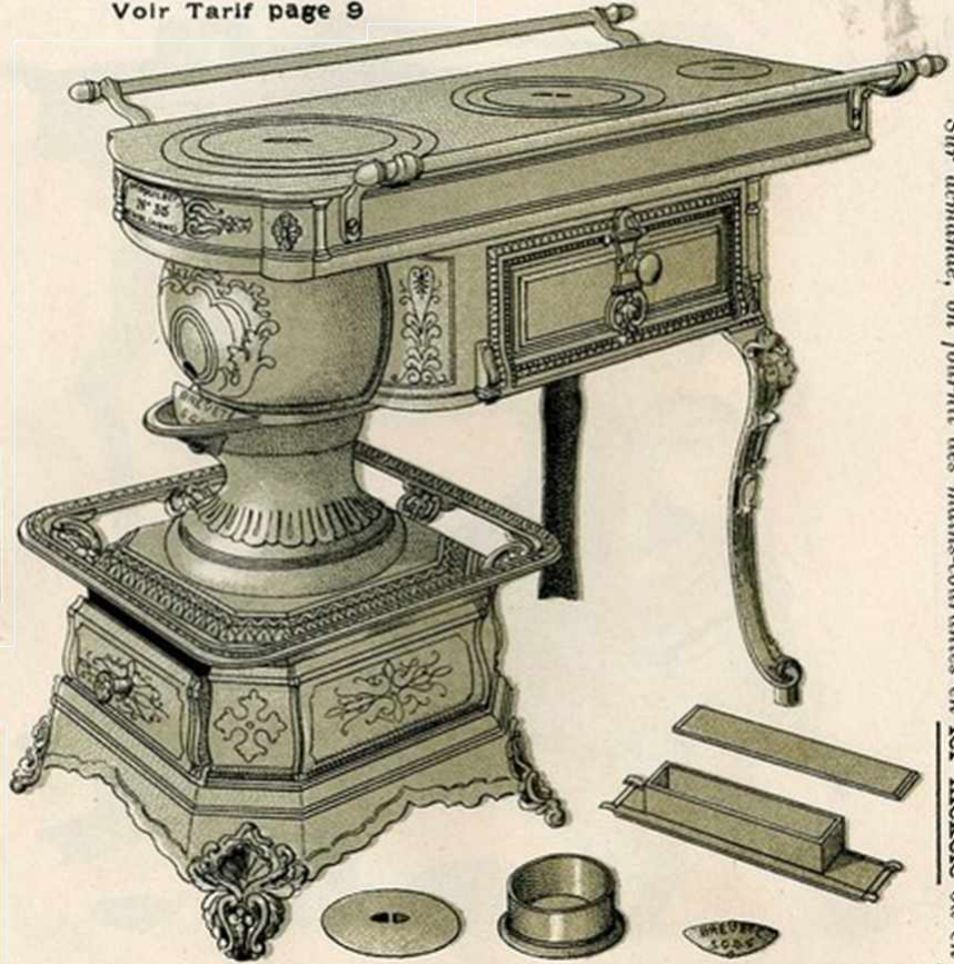
Tampon de buse ronde. Buse ronde de dessus. Papillon.
