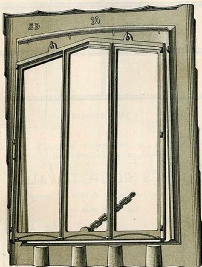
A TROIS VITRES
